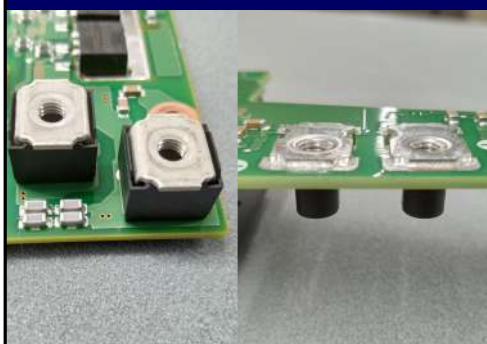
基板間接続
