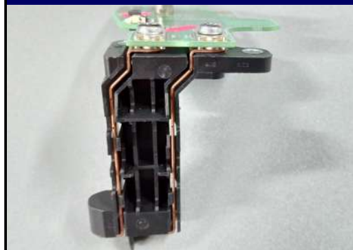
バスバー接続 Busbar connection
